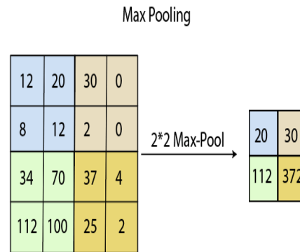
Fig. 4. Pooling Layer
